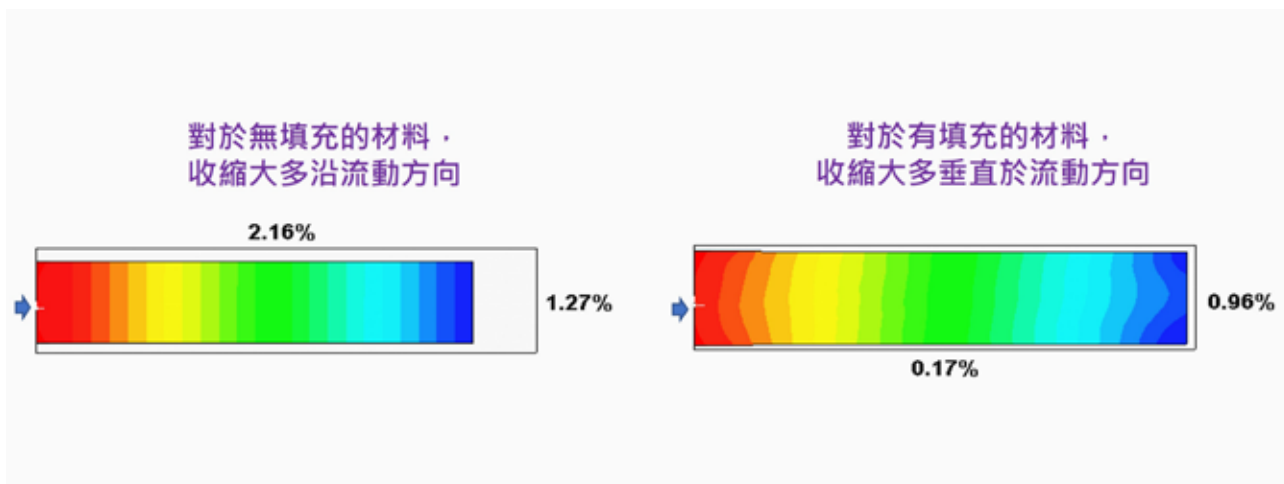
圖 3：無填充與有填充材料的收縮取向差異
