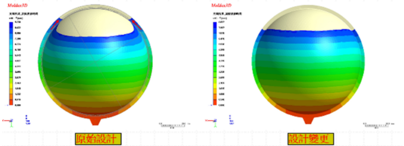
圖 9：設計變更前後流動 80% 對比
