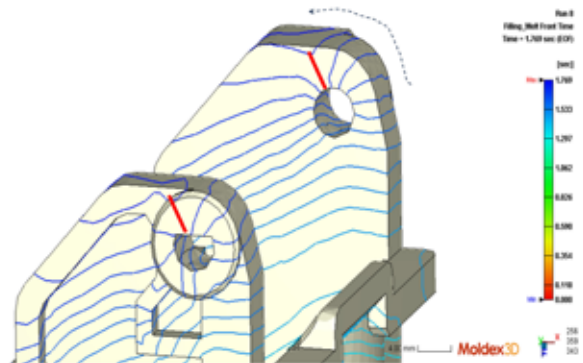
圖 8：由圖中了解其結合線有移到孔洞較寬區
