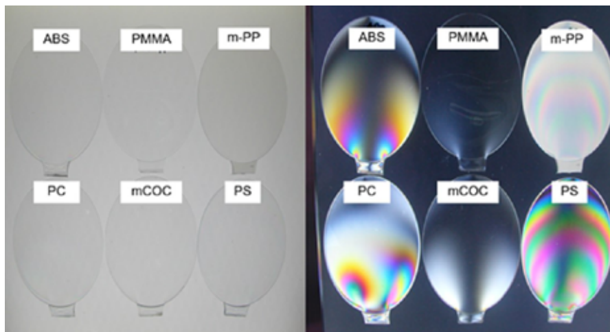
圖 2：同工藝、不同材料下的應力分布
