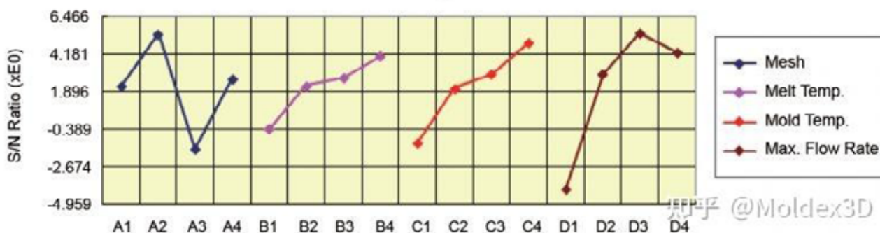
圖 4：充填階段的剪切應力分布之信號 zz 噪聲比
