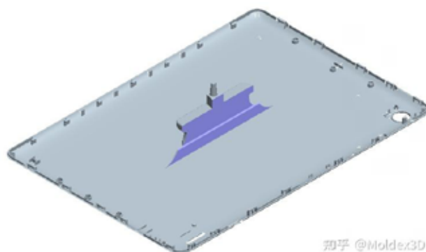
圖 2：原始澆口設計
