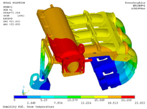
圖 9：進氣歧管的模態分析
