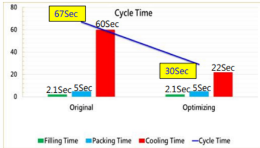
圖 16：改善前後 Cycle Time 對比
