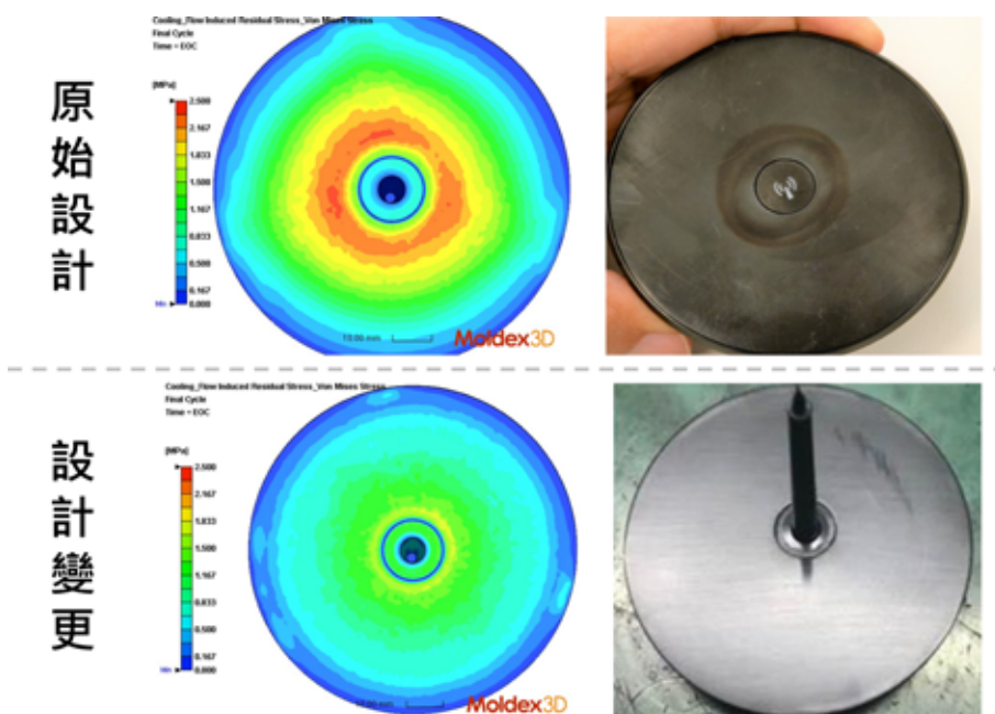
圖 4：以模流分析解決產品應力痕問題。上半部為原始設計；下半部為設計變更
