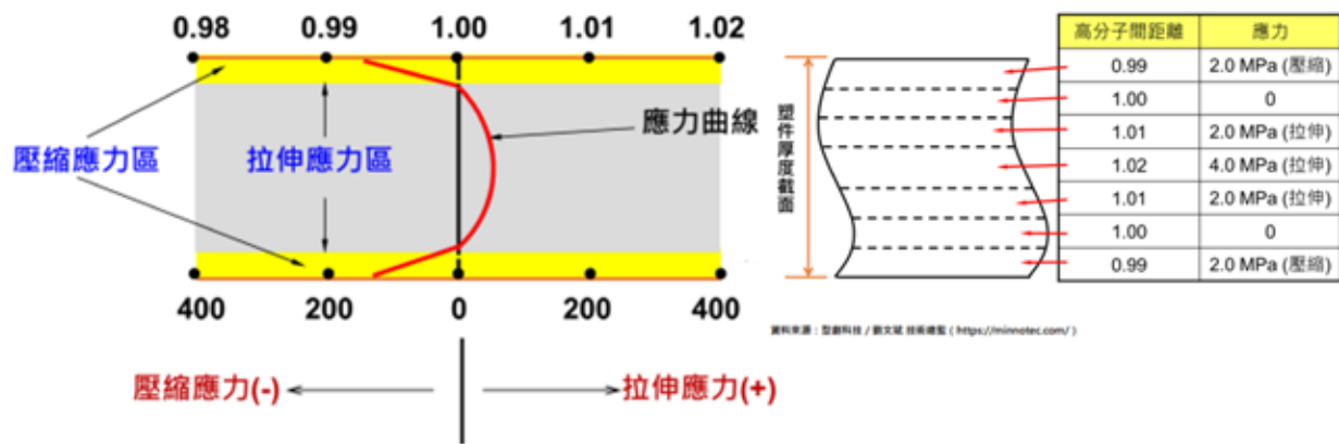
圖 1：塑件冷卻結束後的高分子間距與應力狀態
