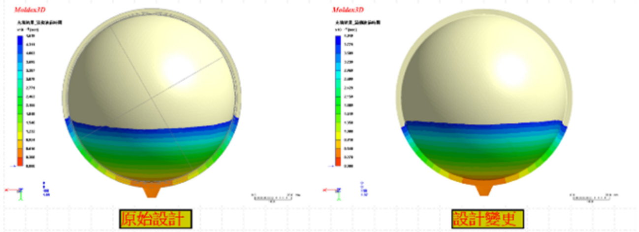
圖 7：設計變更前後流動 40% 對比
