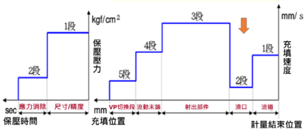
圖 2：充填速度與保壓壓力設定參考
