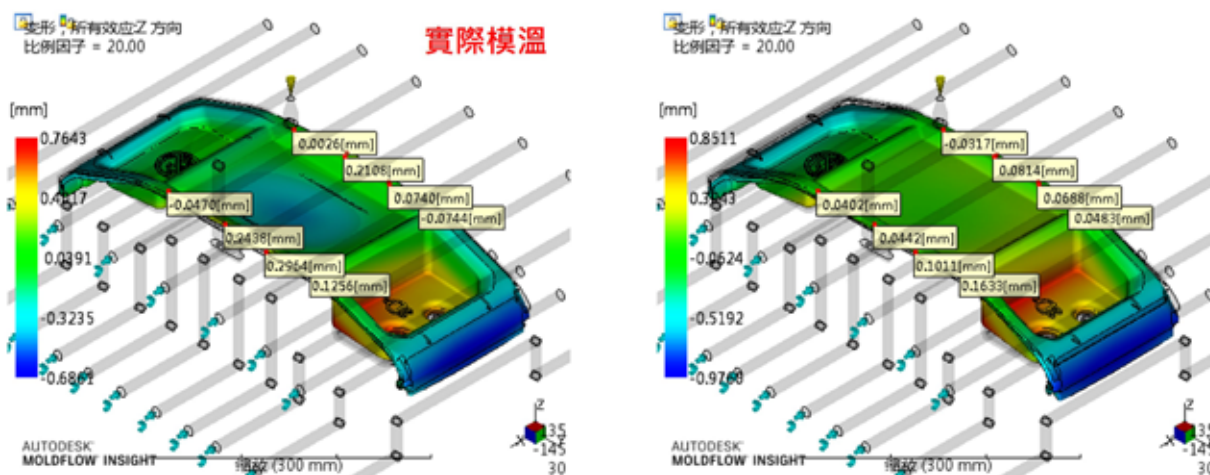
圖 2：通過優化模溫改善冷卻不均引起的變形
