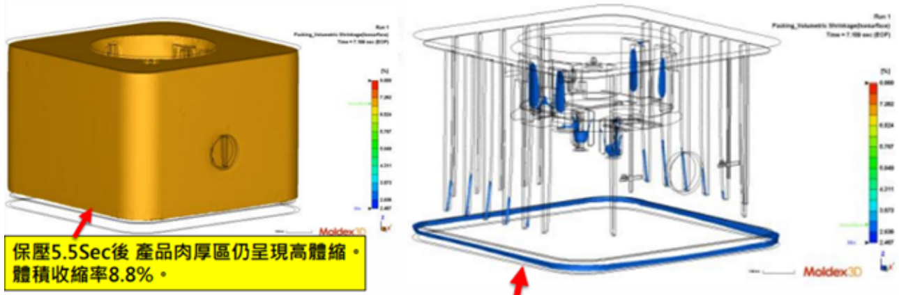
圖 4：厚薄區域的體積收縮率結果
