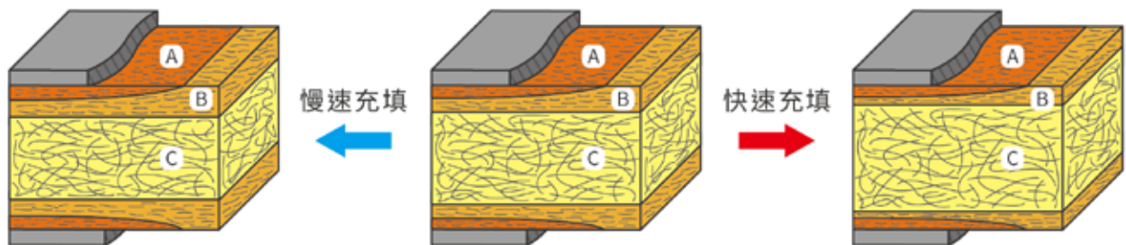
圖 3：充填速率對高分子鏈排向的影響
