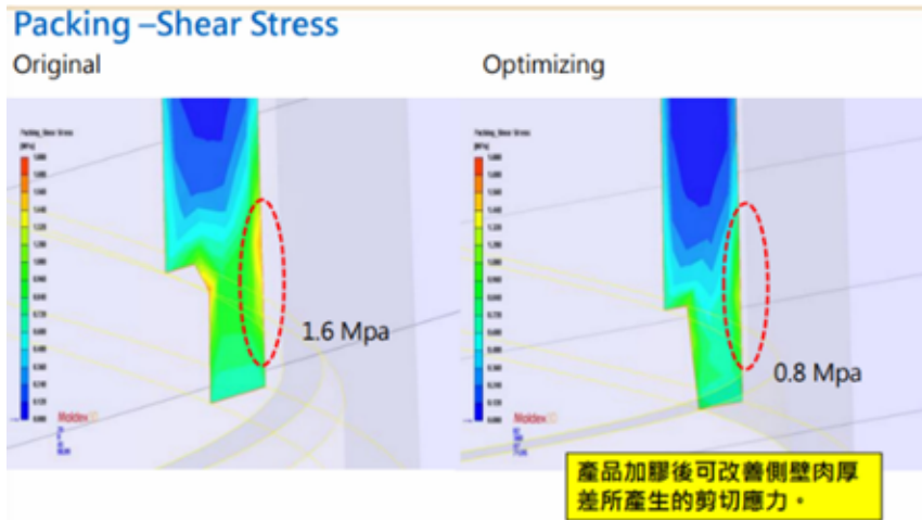
圖 9：加膠前後剪切應力結果對比
