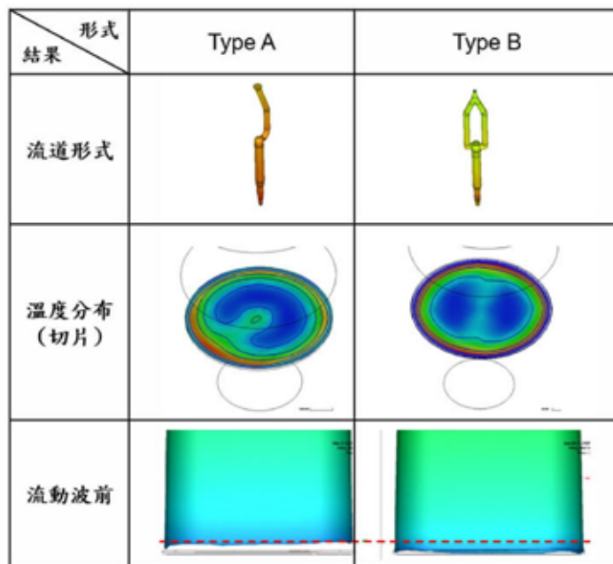
圖 2：不同流道形式之溫度與流動波前比較
