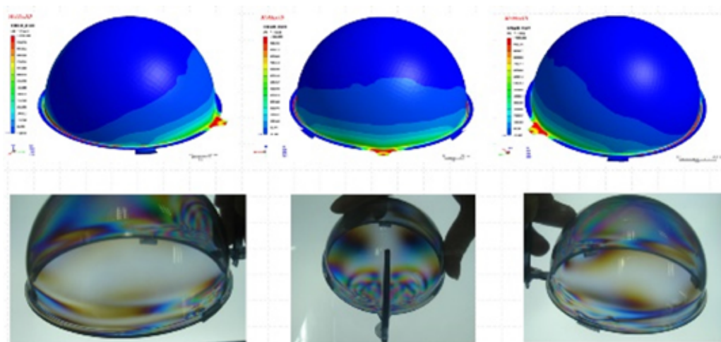
圖 5：剪切率結果及產品實際應力分布圖
