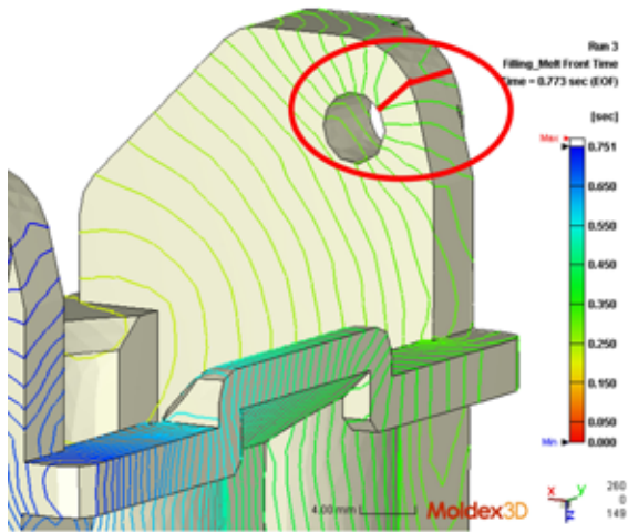
圖 5：射出波前等位線看到結合線在孔洞狹窄區
