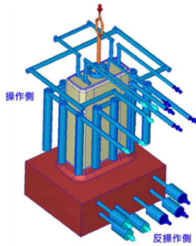
圖 6：冷卻水路設計
