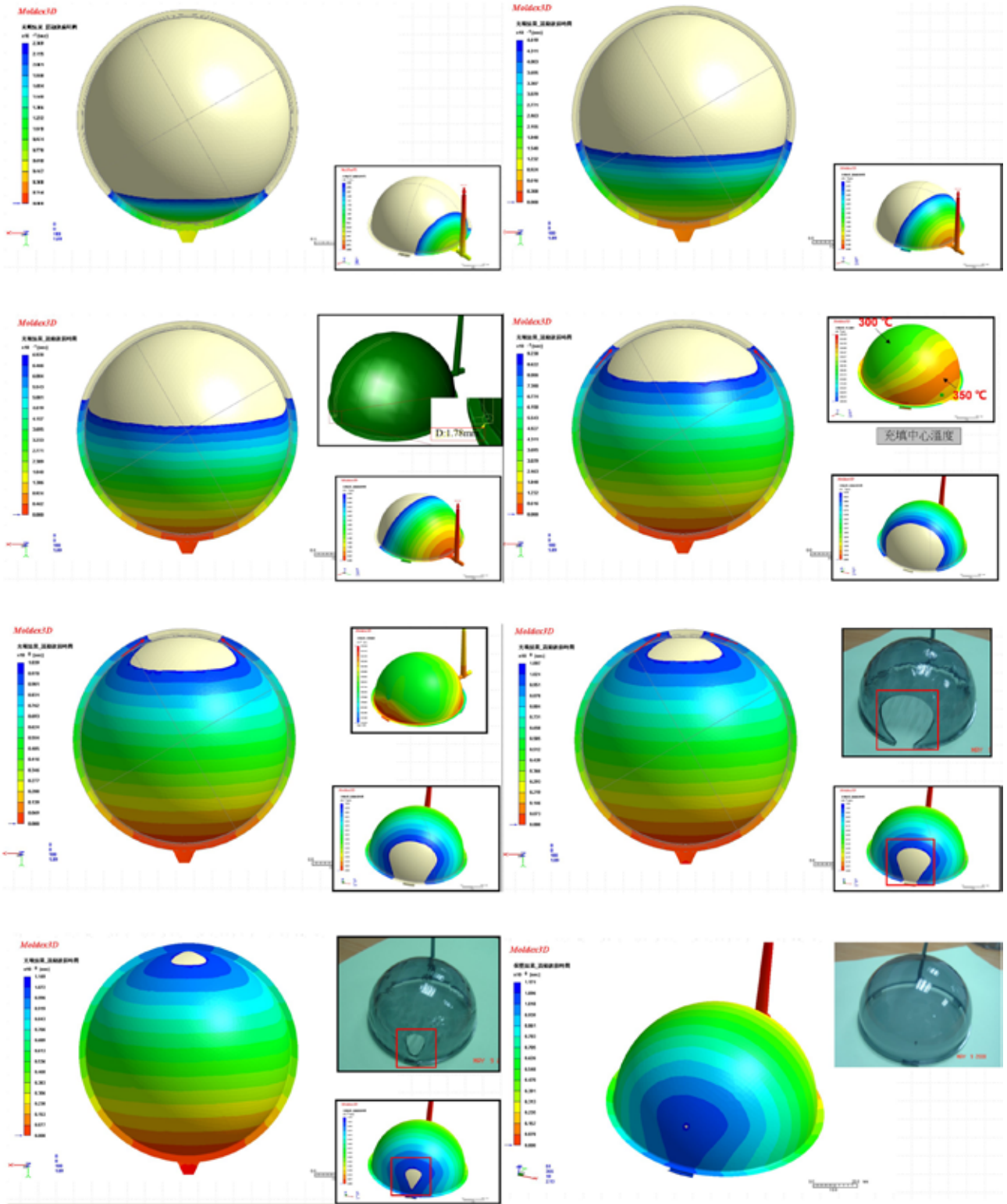
圖 3：流動波前 20%~99.9% 結果
