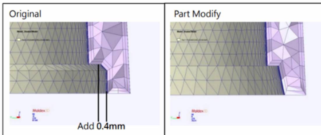
圖 8：美工縫加膠設計
