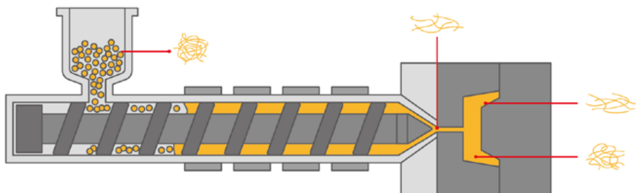
圖 1：射出成型過程中微觀下塑膠高分子鏈的形態變化
