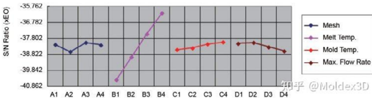
圖 5：充填階段的進澆口射出壓力值之信號噪聲比
