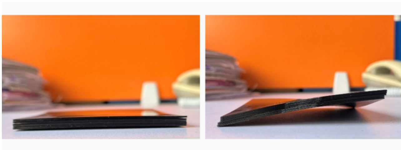
圖 4：左為金陽低翹曲 PBT-GF30 材料；右為普通 PBT-GF30 材料
