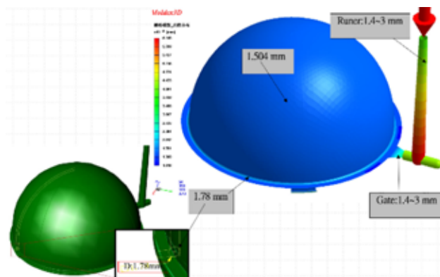
圖 2：產品及流道肉厚分布
