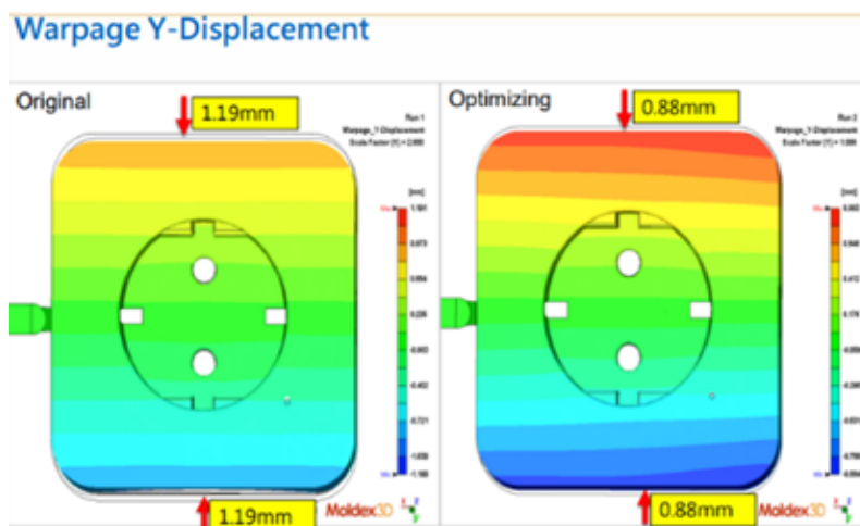
圖 14：Y 方向翹曲結果線性收縮率對比
