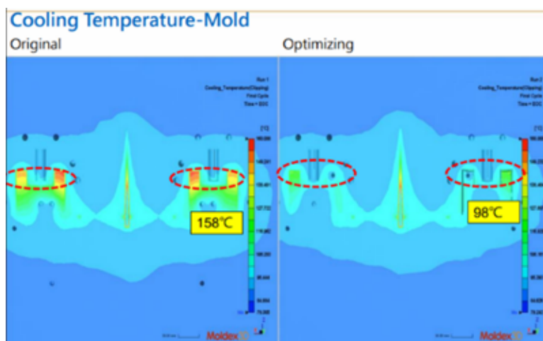
圖 12：改善前後模具溫度結果對比
