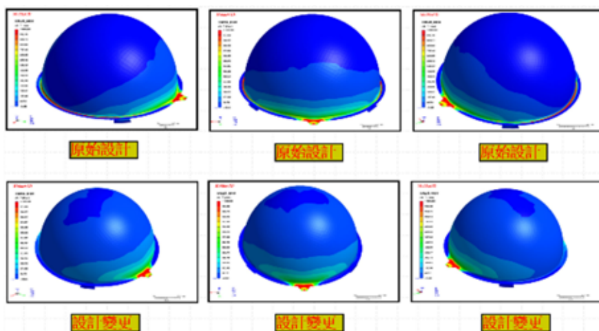
圖 12：改善前後剪切率結果對比
