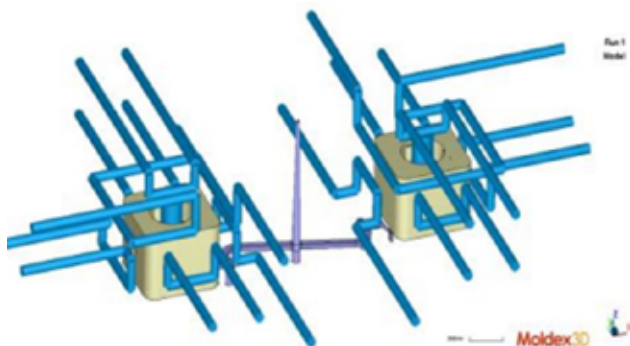
圖 1：塑料射出成型部件
