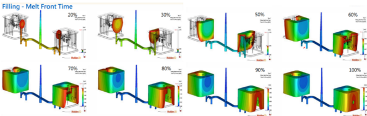
圖 3：流動波前 20%~100%
