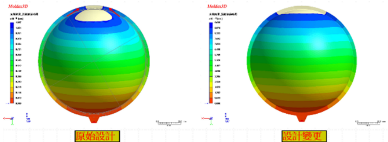
圖 10：設計變更前後流動 95% 對比
