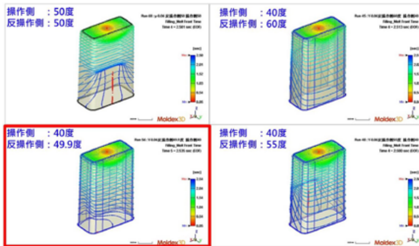
圖 7：公模仁位移 0.06mm 搭配模溫控制對流動結果影響
