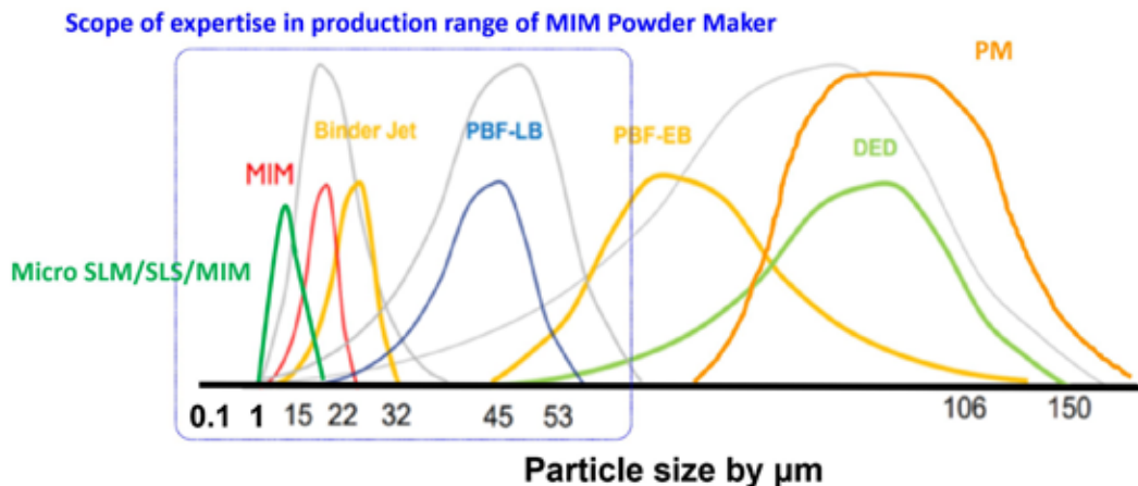
圖 2：目前 PM、MIM 和 MAM 金屬粉末使用的粒徑分佈圖。本圖由 Dr. Q 修改自英國山特維克公司提供的原圖。(這裡並沒有考慮粉末的形狀)
