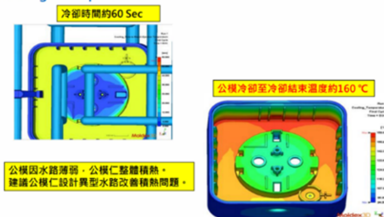
圖 6：公模冷卻時間及溫度結果
