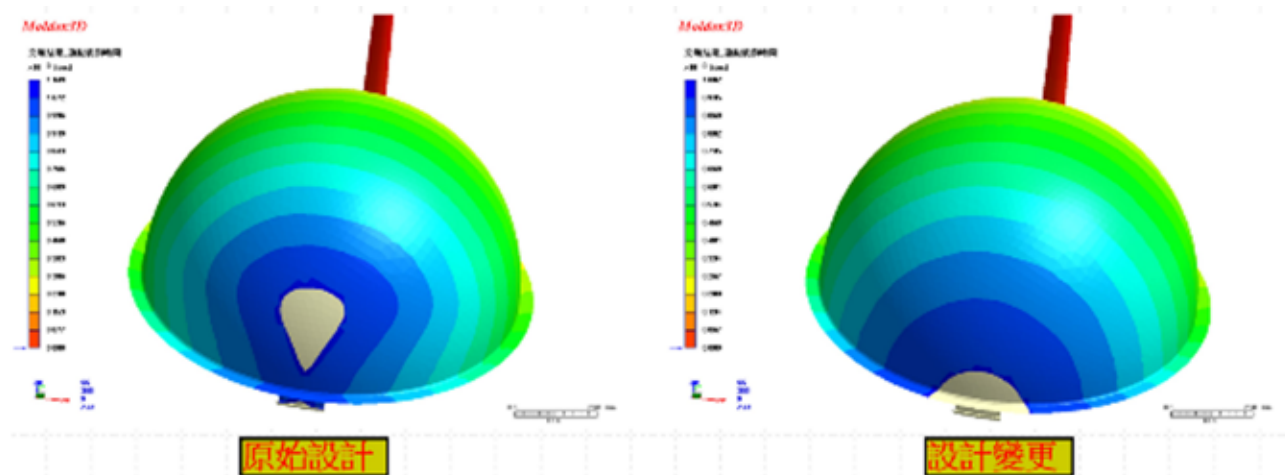
圖 11：設計變更前後包封位置
