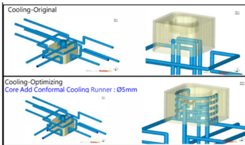
圖 7：異形水路設計方案
