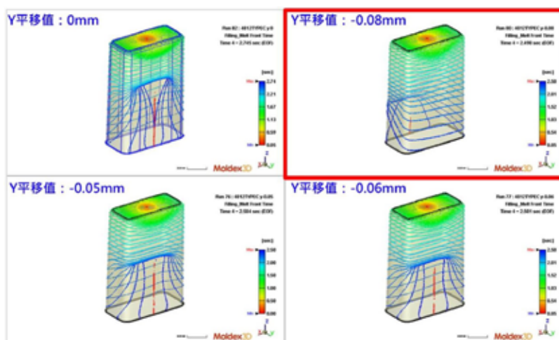
圖 5：公模仁位移對流動結果影響
