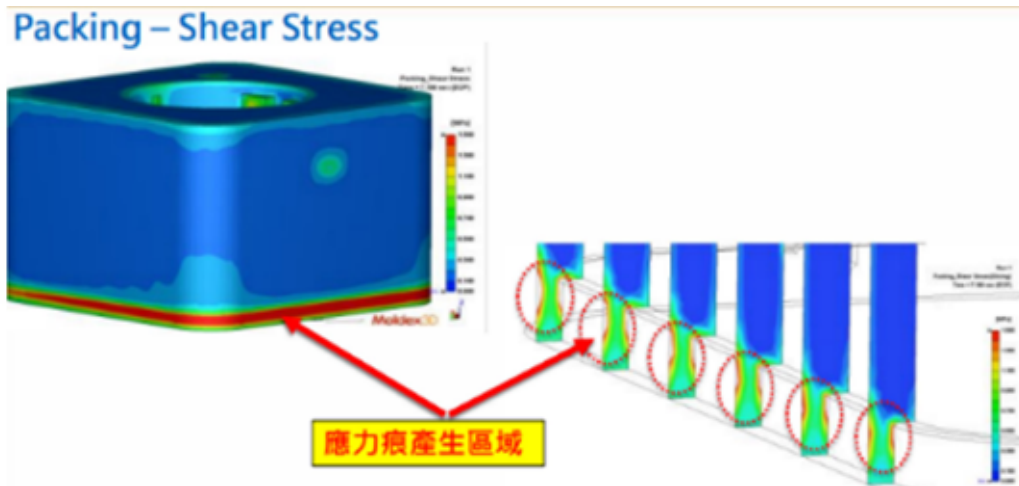
圖 5：剪切應力結果
