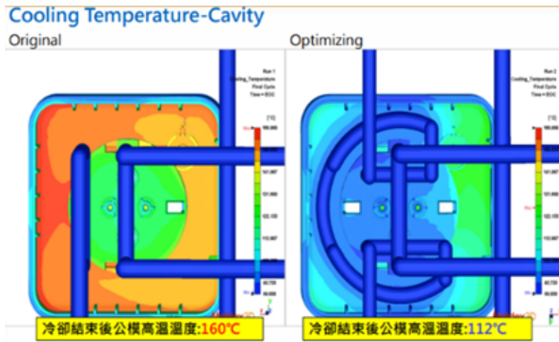
圖 10：改善前後公模高溫溫度對比
