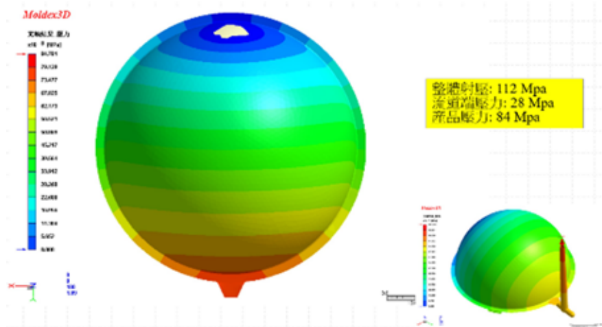
圖 4：充填壓力分布
