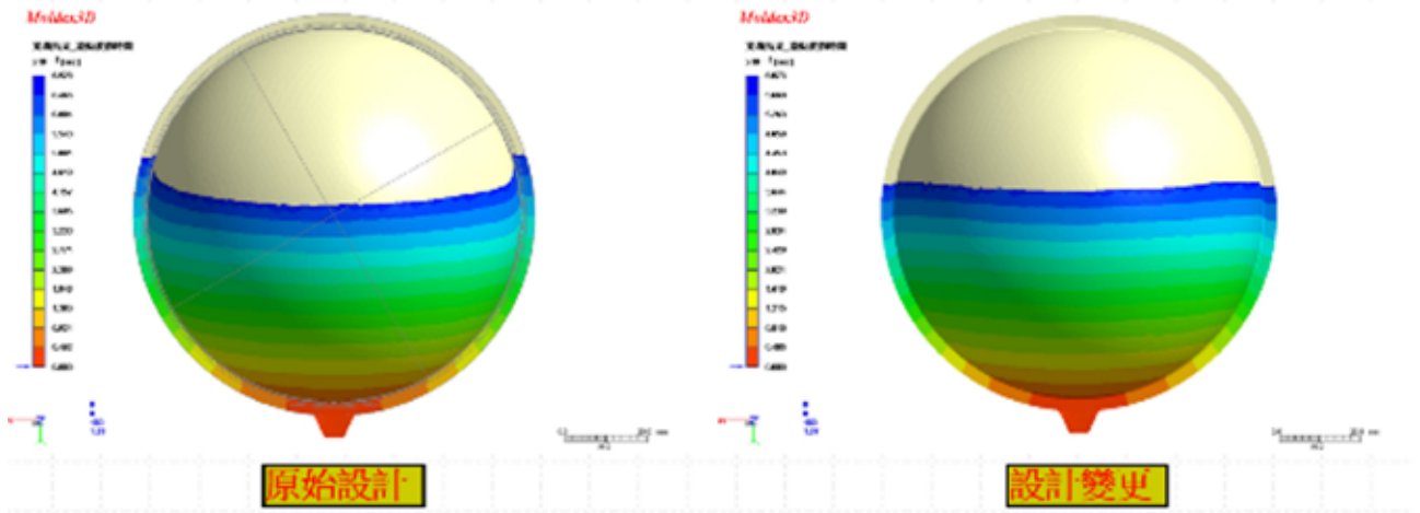
圖 8：設計變更前後流動 60% 對比
