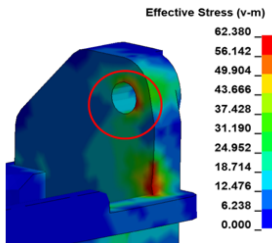
圖 3：轉軸強度設計——結構強度分析
