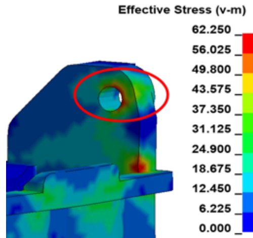
圖 6：初版評估進膠位置，結合線位置位於軸孔受力位置，轉軸孔有斷裂風險
