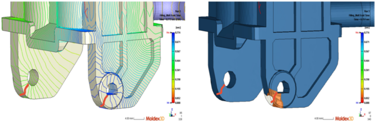
圖 4：模流分析模穴充填體積 95% 對應軸孔產生結合線位置
