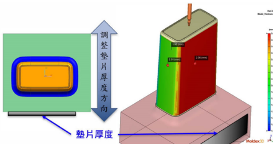
圖 4：公模仁往 -Y 方向平移
