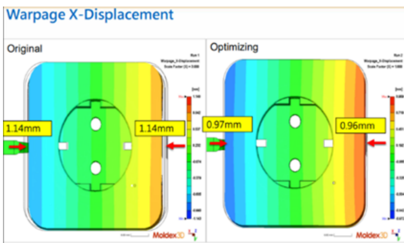
圖 13：X 方向翹曲結果線性收縮率對比
