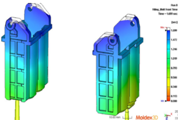
圖 7：設計變更後局部厚度改變流動波前
