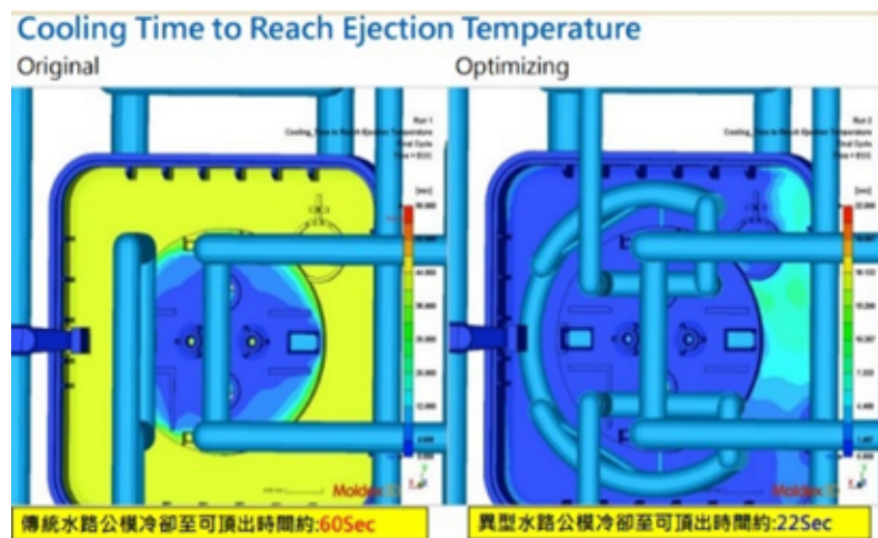
圖 11：改善前後公模冷卻至頂出時間對比
