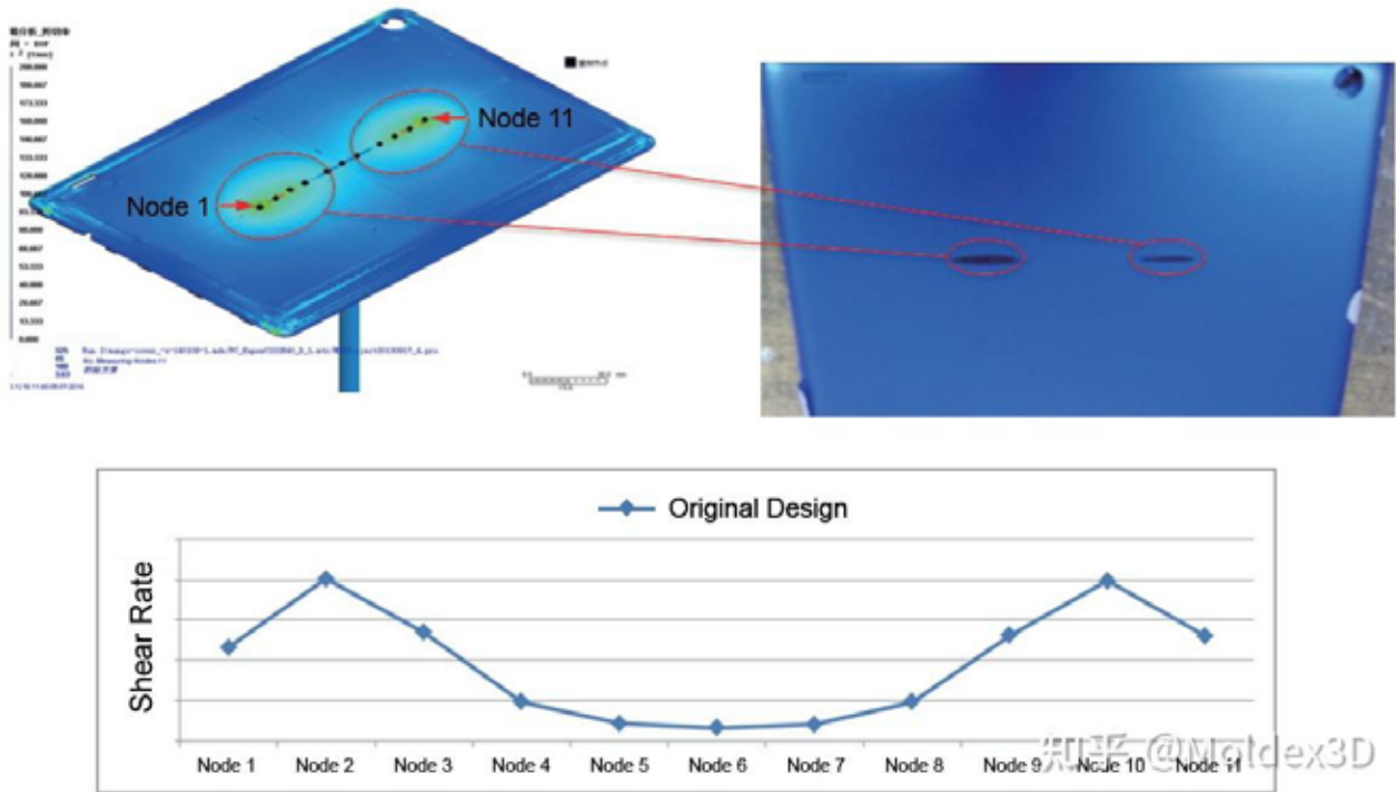
圖 3：原始設計在充填階段的剪切速率分析結果
