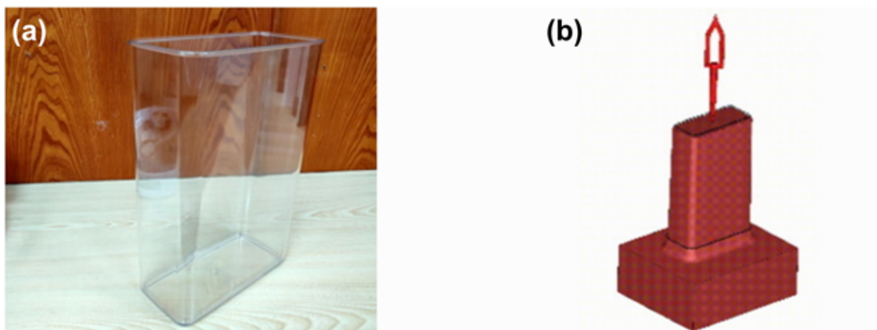
圖 1：易撥罐之罐身產品。(a) 罐身；(b) 公模仁幾何
