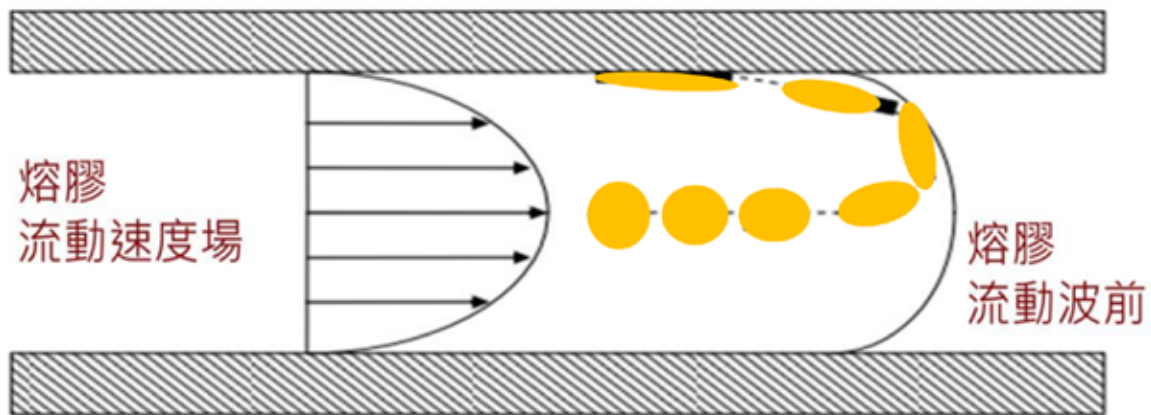
圖 2：塑料熔膠受噴泉流引導的高分子鏈形態變化與排向分布
