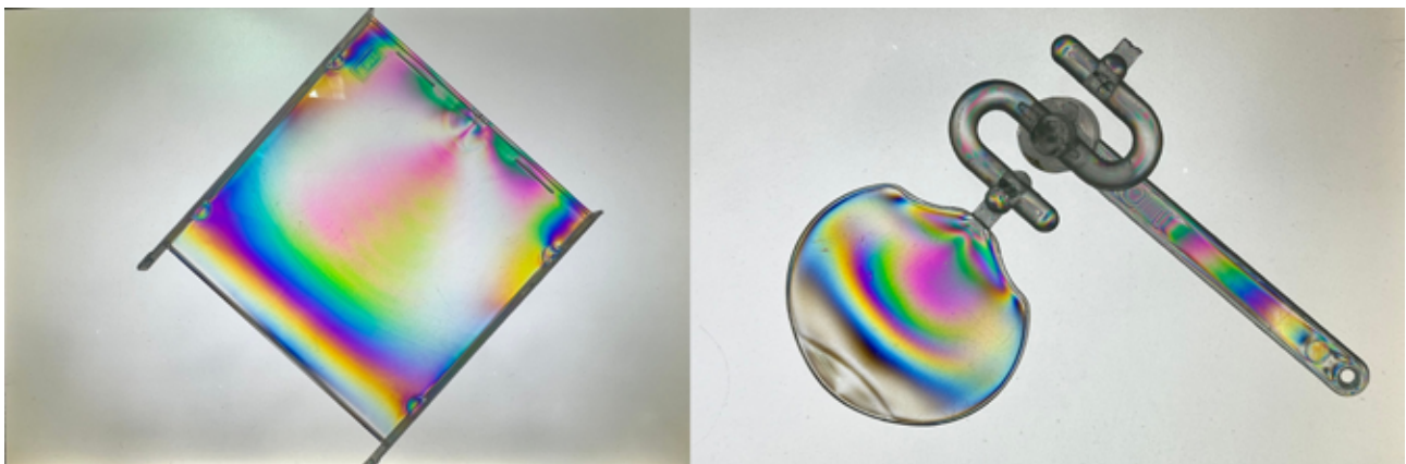
圖 3：產品進澆處及角落有較高殘留應力
