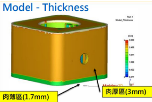
圖 2：產品肉厚差異區域產生應力痕
