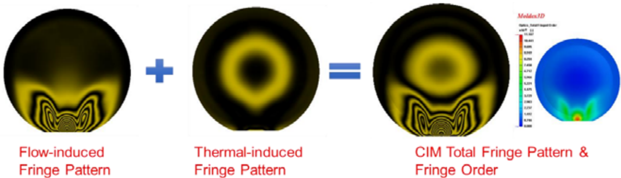
圖 2：流動導致與熱導致殘留應力
