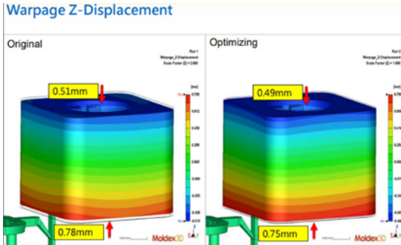
圖 15：Z 方向翹曲結果線性收縮率對比
